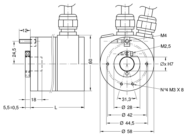
ASC58/AMC58
